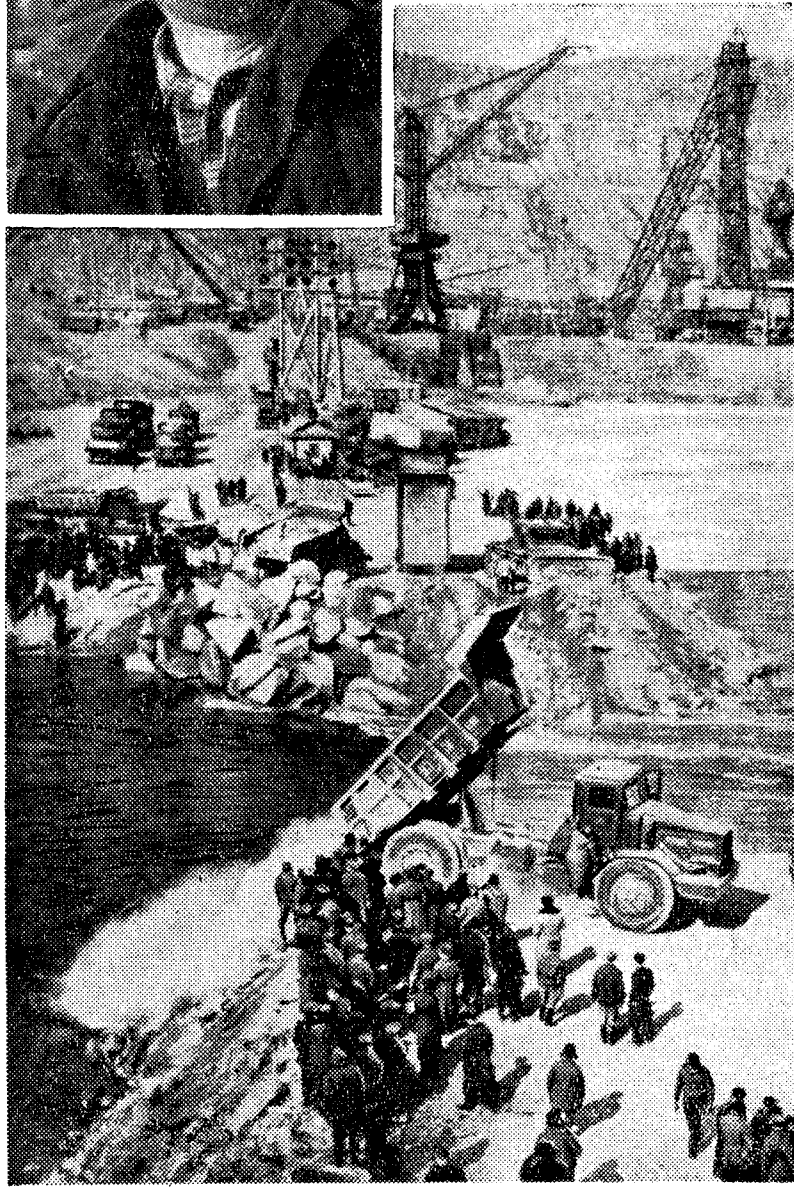
ДВНГОРСК. День перекрытия великого Енисея стал настоящим праздником, триумфом труда строителей Красноярской ГЭС. На нижнем снимке: самосвалы сбрасывают бетонные глыбы в проран. Вверху — водитель 25-тонного самосвала Леонид Назимко. Он первым в день перекрытия вступил в борьбу с Енисеем. Фото В. Соболева и Ю. Бармина. (ТАСС). (Принято по фототелеграфу).
